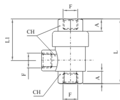
VES: VÁLVULA DE RETENCIÓN HxHxH CILÍNDRICA
