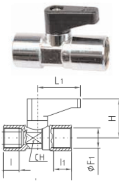
VHH-C: VÁLVULA BOLA MINI COMPACTA HxH
