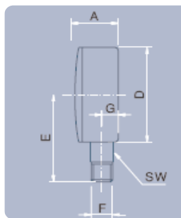
MR40 - MR50 - MR63: MANÓMETRO CAJA PLÁSTICO SALIDA RADIAL -20 +60°C P >2,5 Bar >1,6 Bar (bajo pedido) Grado P. IP43
