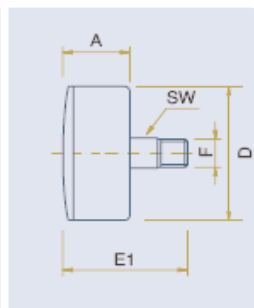
M40 - M50 - M63: MANÓMETRO CAJA PLÁSTICO SALIDA POSTERIOR -20 +60°C P >2,5 Bar >1,6 Bar (bajo pedido) Grado P. IP43
